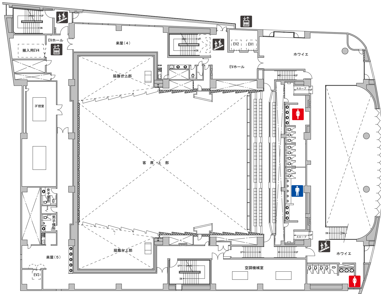
3階平面図
