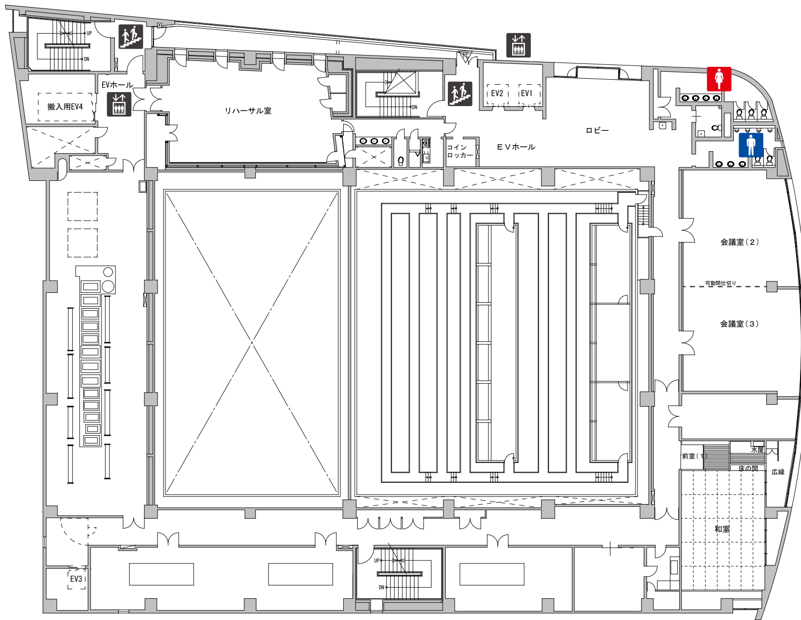
4 階 平 面 図
